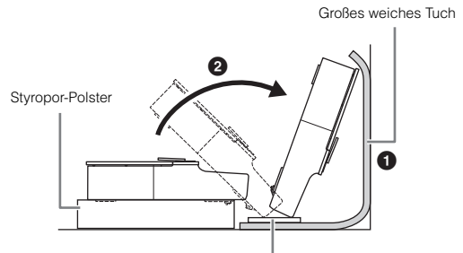
Schutzpolster
