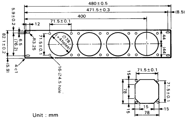
Fan panel
