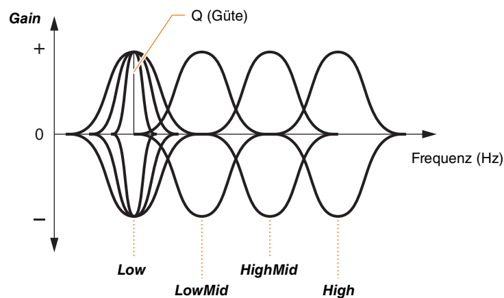
Vier EQ-Bänder
